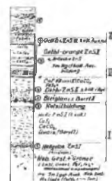
Fig 10a: Profil im 6. Verhau (Lgd-Trum des Haupterzanges (Allg-Str. d. Innenfüllung - u. Neb-Gest-Streichen)
